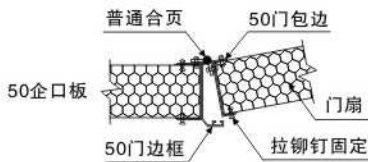
普通门大样
