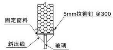
固定窗节点
