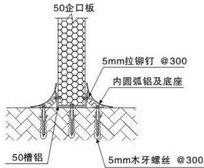
地面与墙板节点大样 (净化)
