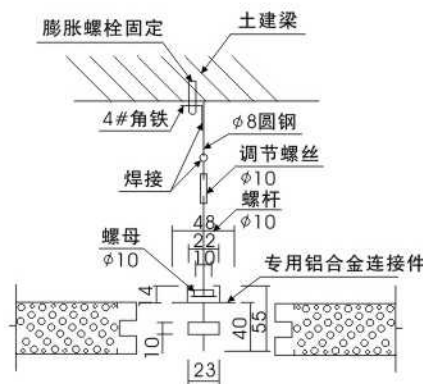
板与板连接（2）
