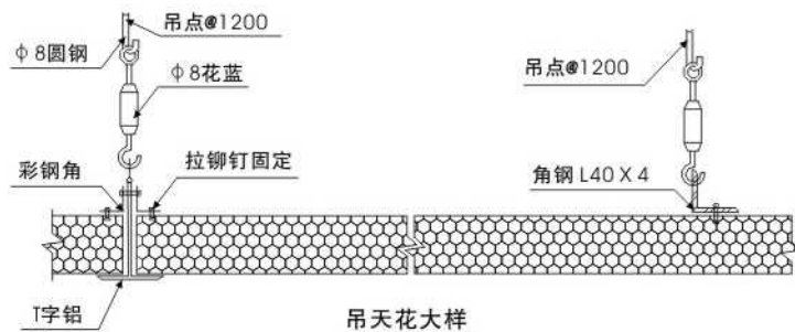
吊天花大样
