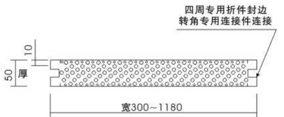
手工板（中字形）：用于围护隔断、吊顶
