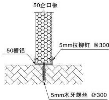
地面与墙板节点大样
