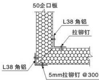
普通转角大样
