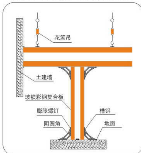
丁字接点:
