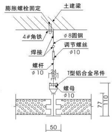
板与板连接（3）
