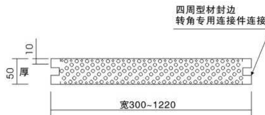
手工板（中字形）：用于围护隔断
