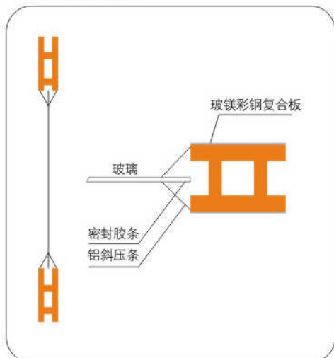
墙面接点:
