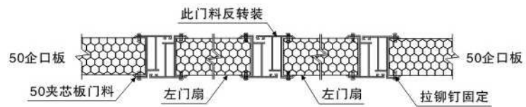
双掩门大样
