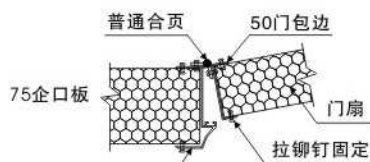
75系列门料
