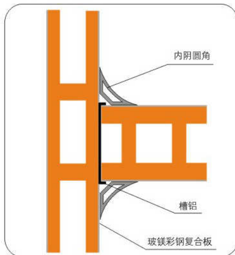
与地面接点:
