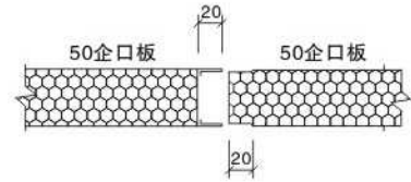
企口板拼缝节点
