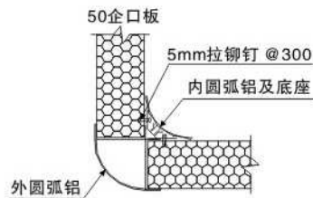
净化转角大样
