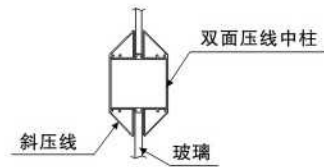
固定窗中柱节点
